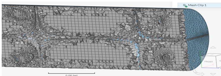
Рисунок 2 - Расчетные сетки (грубая, средняя, мелкая)
