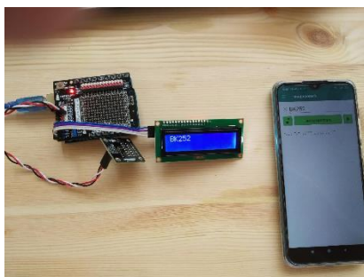
Рисунок 4 - Дешифратор азбуки Морзе в процессе его работы
