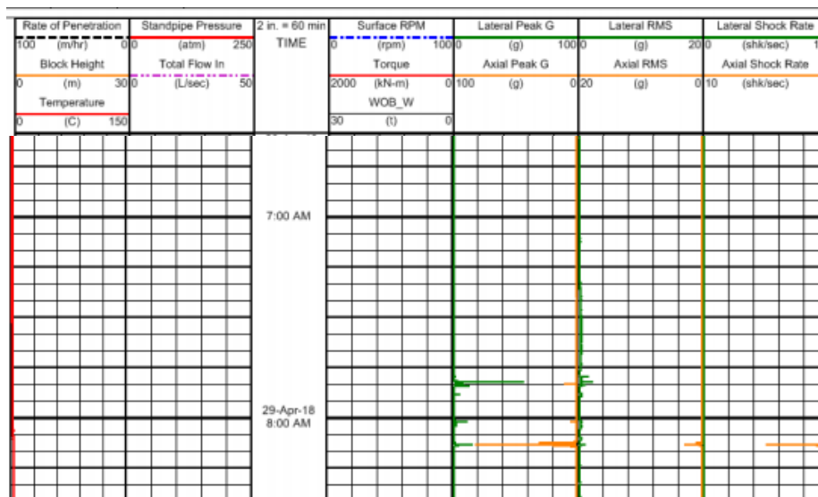
Рисунок 5 – Анализ вибраций в интервале пиковых значений по оси X и Y Имлорского месторождения
