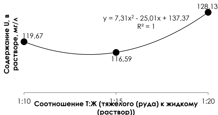
Рисунок 4 - Извлечение урана при плотности раствора тяжелого (руда) : к жидкому (раствор) и влияние на скорость окисления железа штаммом бактерий Acid. ferrooxidans
