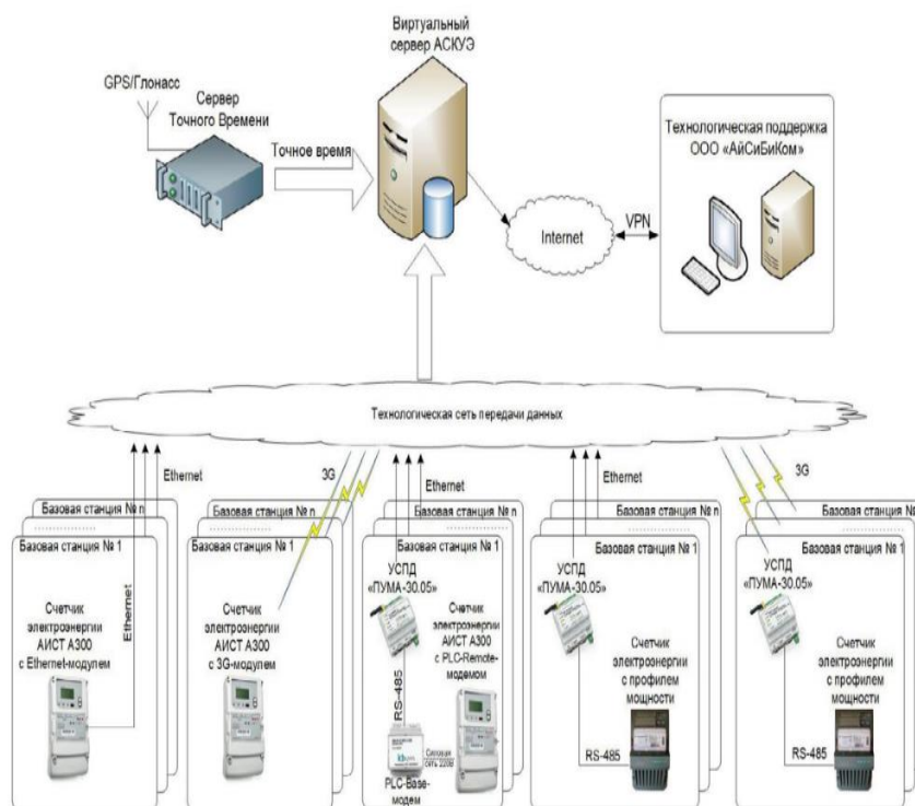
Рисунок 2 – Схема организации связи
