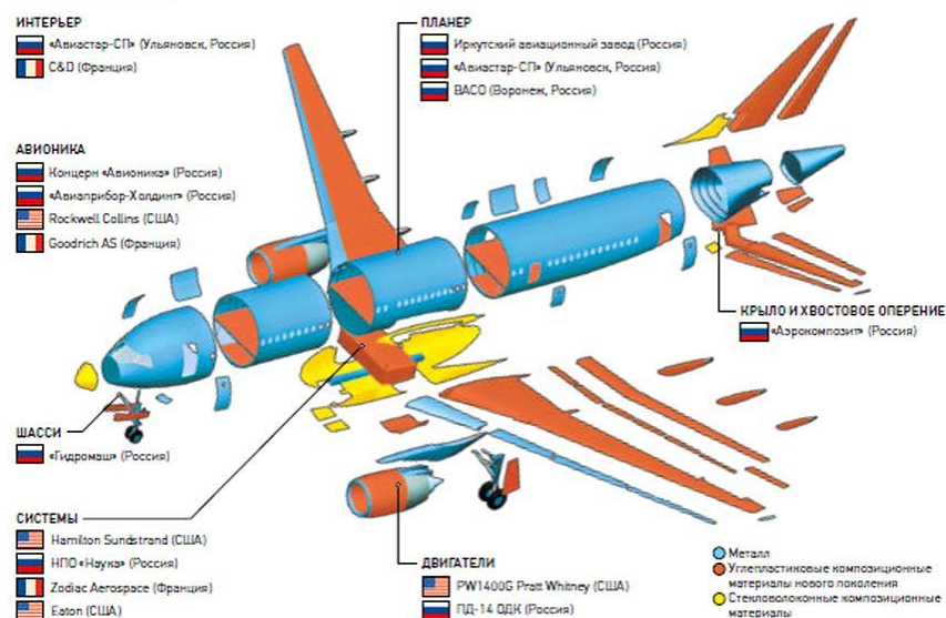
Рисунок 1 - Распределение материалов в конструкции МС-21
