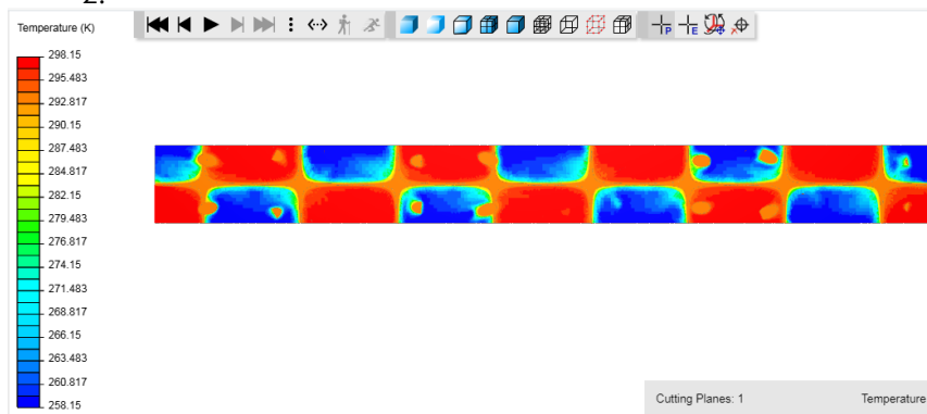
Рисунок 4 - Распределение температуры в продольном сечении
