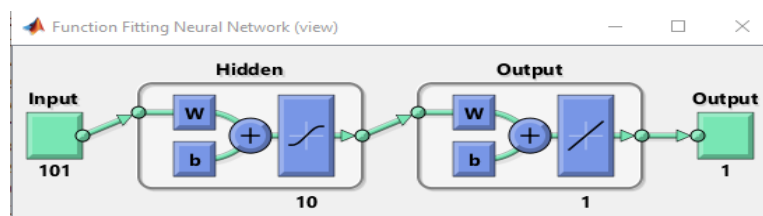
Рисунок 2 — Диаграмма нейронной сети
