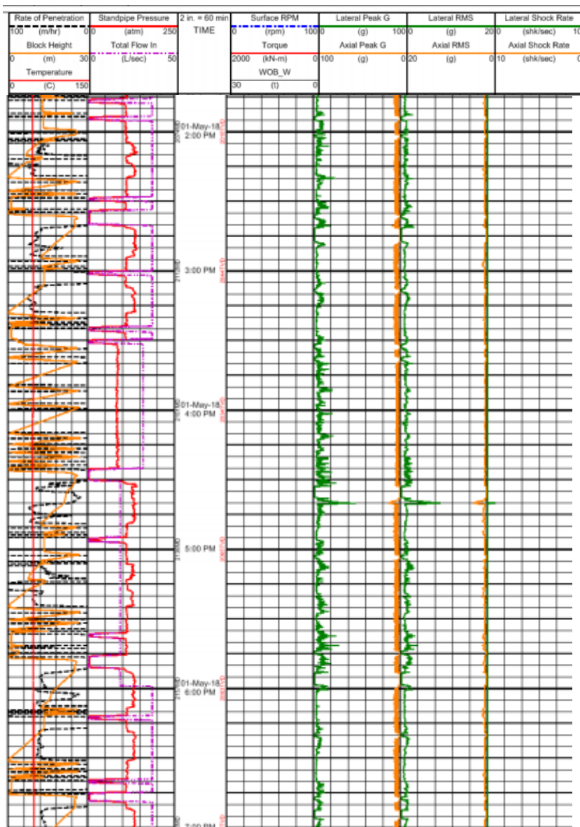
Рисунок 4 – Анализ вибраций в интервале пиковых значений по оси X и Y Имлорского месторождения
