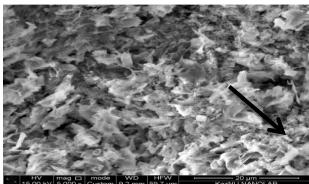
Рисунок 2 - Снимки сканирующего электронного микроскопа руды после длительного времени выщелачивания 2,5% серной кислотой
