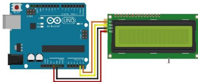
Рисунок 3 - Схема подключения дисплея с использованием I2C
