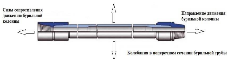
Рисунок 2 - Колебания в поперечном сечении
